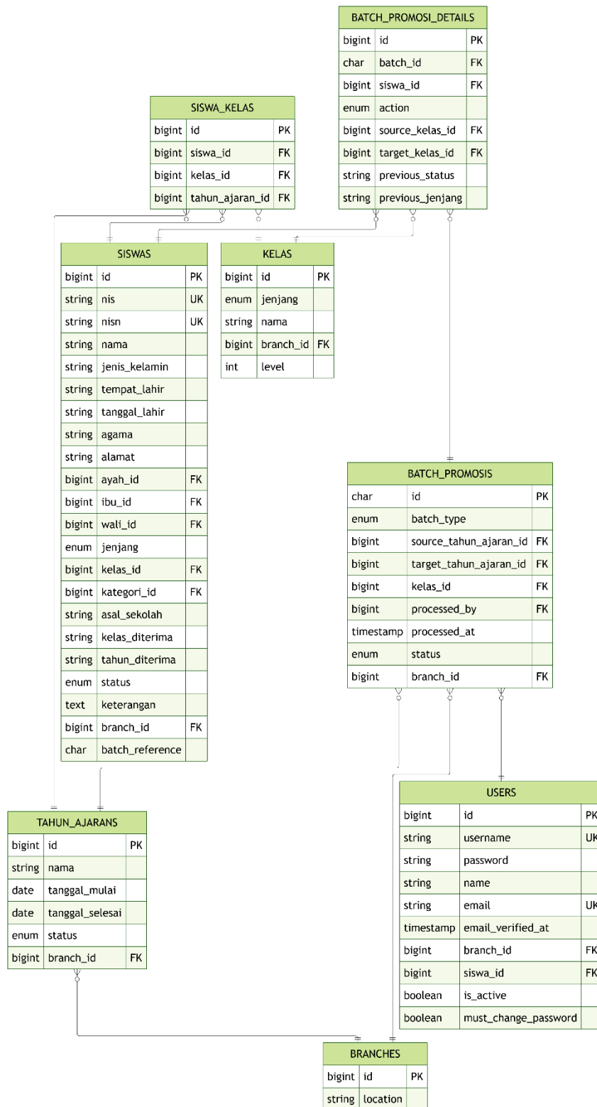
Gambar 3.6. Diagram Relasi Tabel Modul Tahun Ajaran &amp; Kenaikan Kelas
