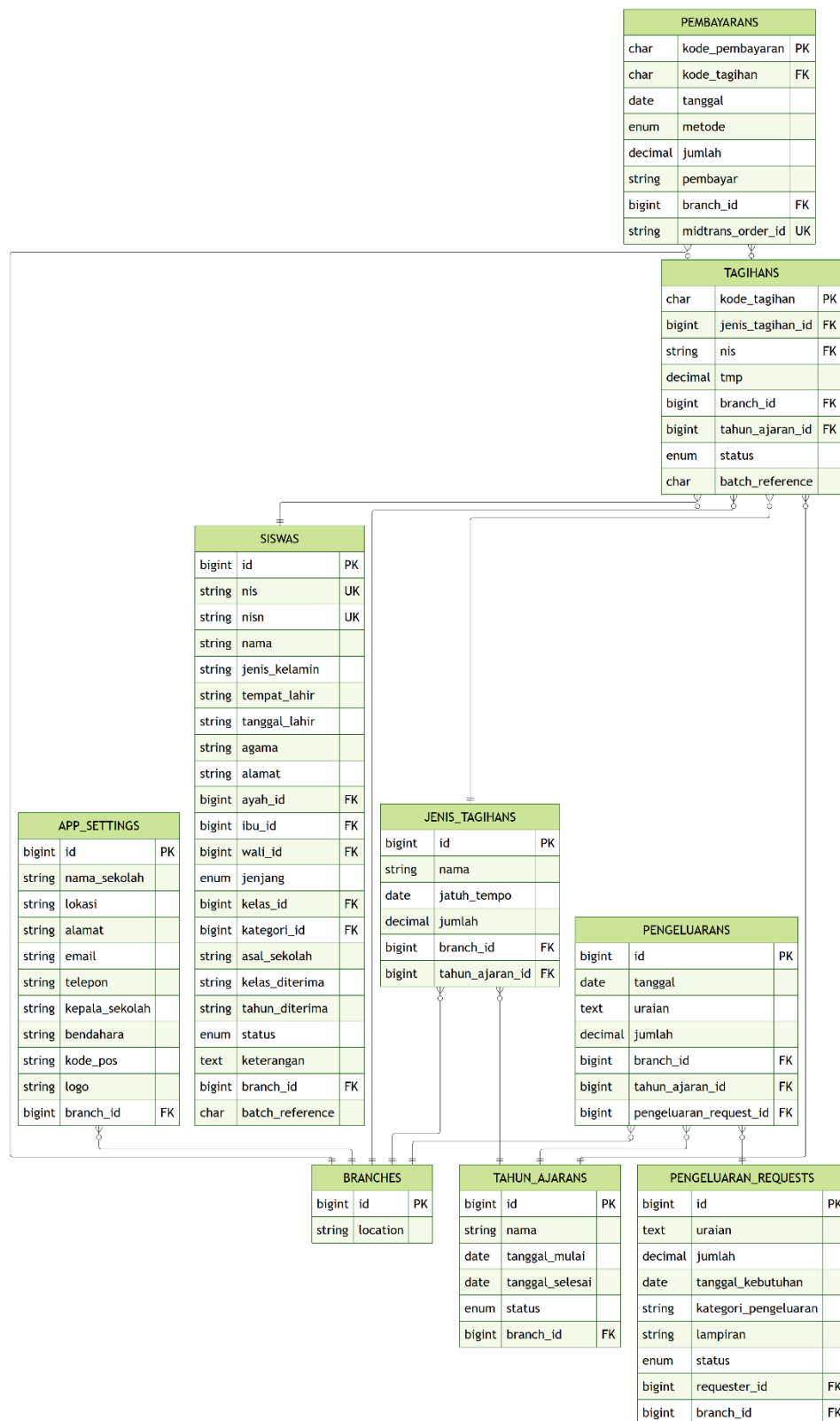
Gambar 3.4. Diagram Relasi Tabel Transaksi Keuangan
