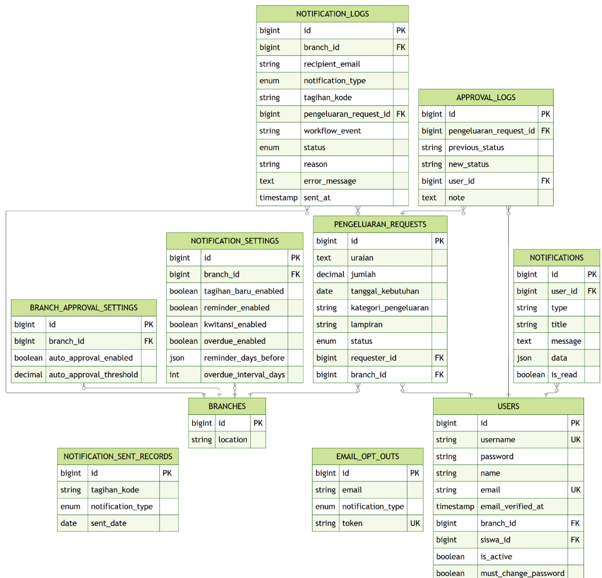
Gambar 3.7. Diagram Relasi Tabel Modul Approval Pengeluaran &amp; Notifikasi
