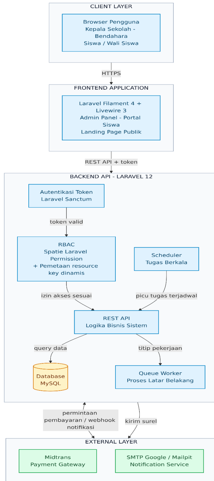
Gambar 3.2. Diagram Arsitektur Sistem
